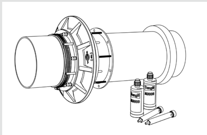
Quadro-Secura® Quick/H
